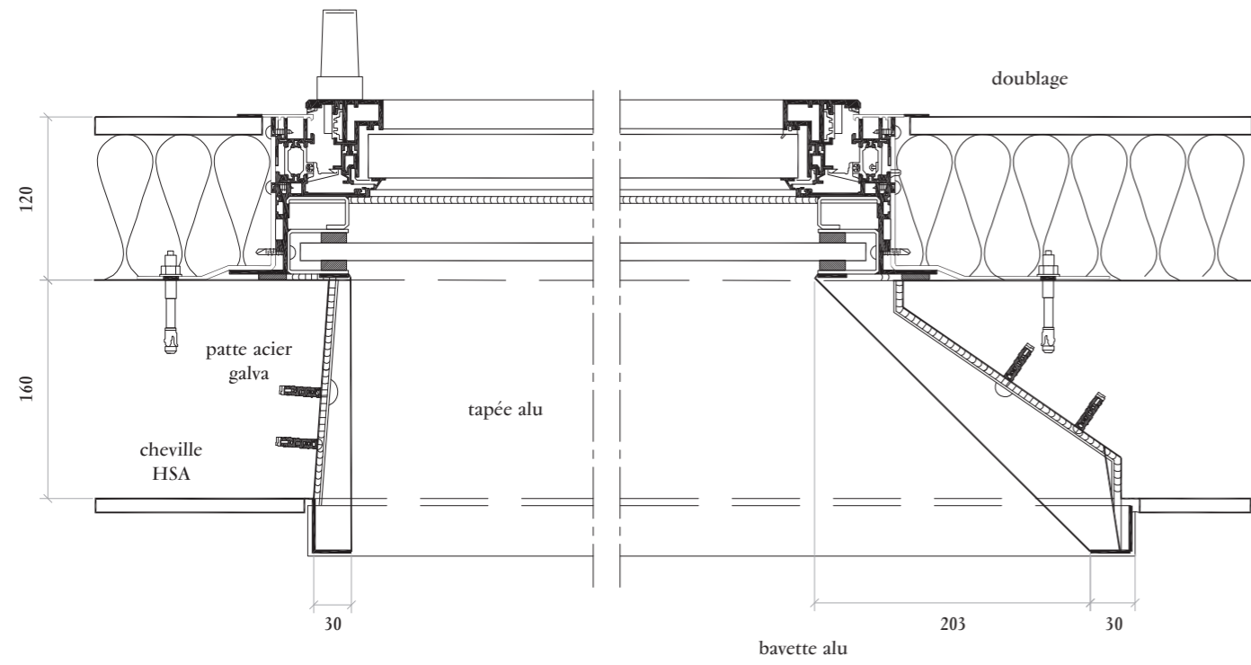
Détail cassette
